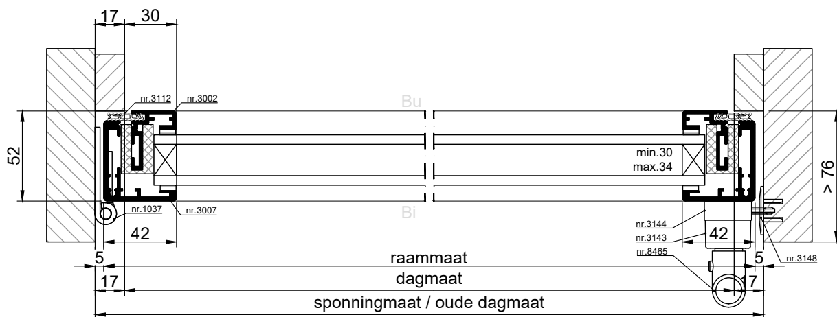
HORIZONTALE DOORSNEDE type AMD-2
