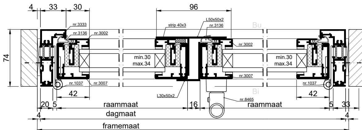
HORIZONTALE DOORSNEDE type AMS-1
