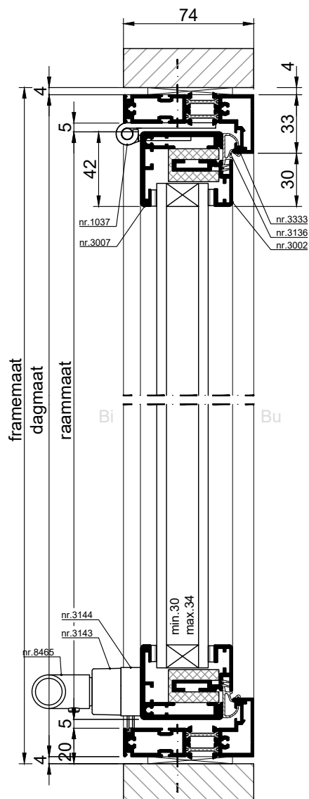
VERTICALE DOORSNEDE type AMK-1
