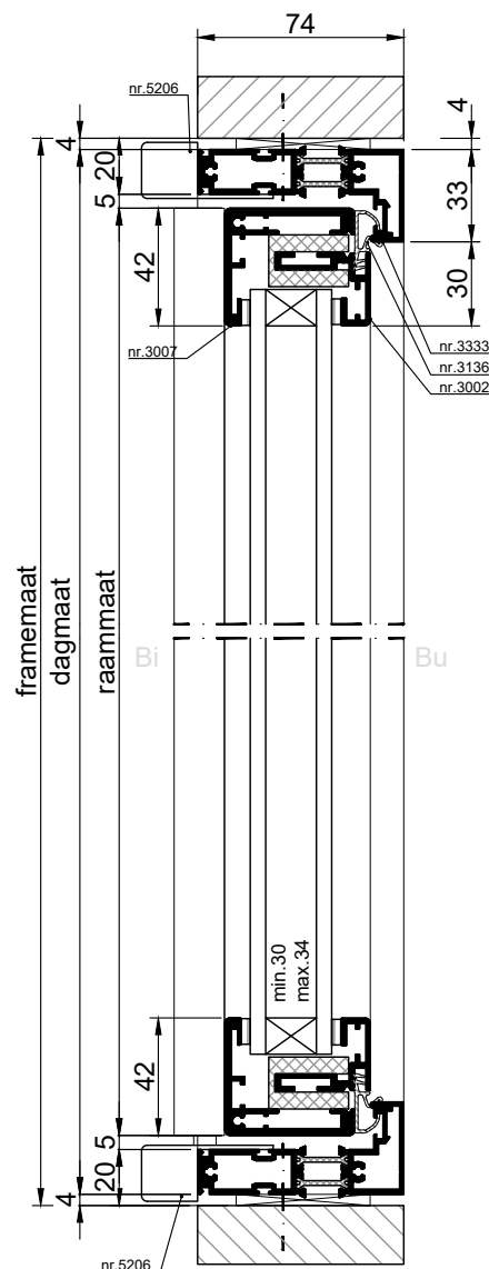
VERTICALE DOORSNEDE type AMS-1
