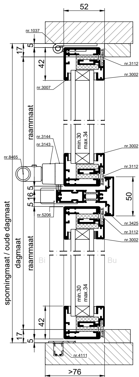
VERTICALE DOORSNEDE type AMC-4
