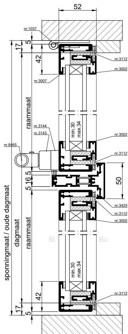
VERTICALE DOORSNEDE type AMC-2
