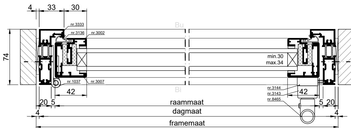
HORizontale Doorsnede type AMC-1
