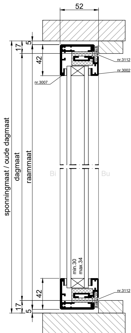
VERTICALE DOORSNEDE type AMD-2
