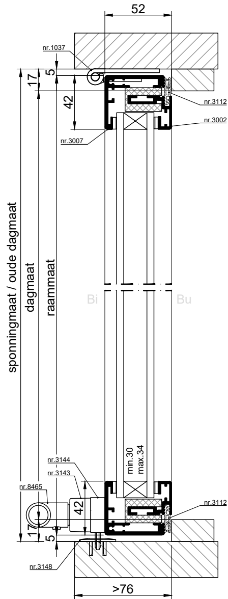
VERTICALE DOORSNEDE type AMK-2
