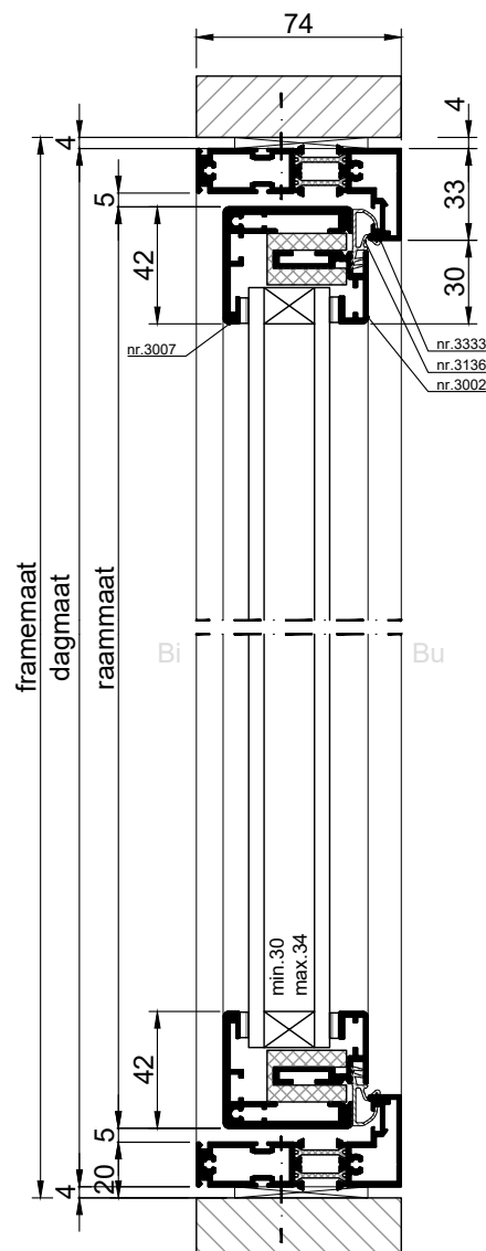
VERTICALE DOORSNEDE type AMD-1
