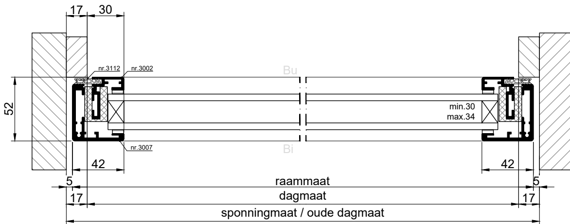
HORIZONTALE DOORSNEDE type AMK-2
