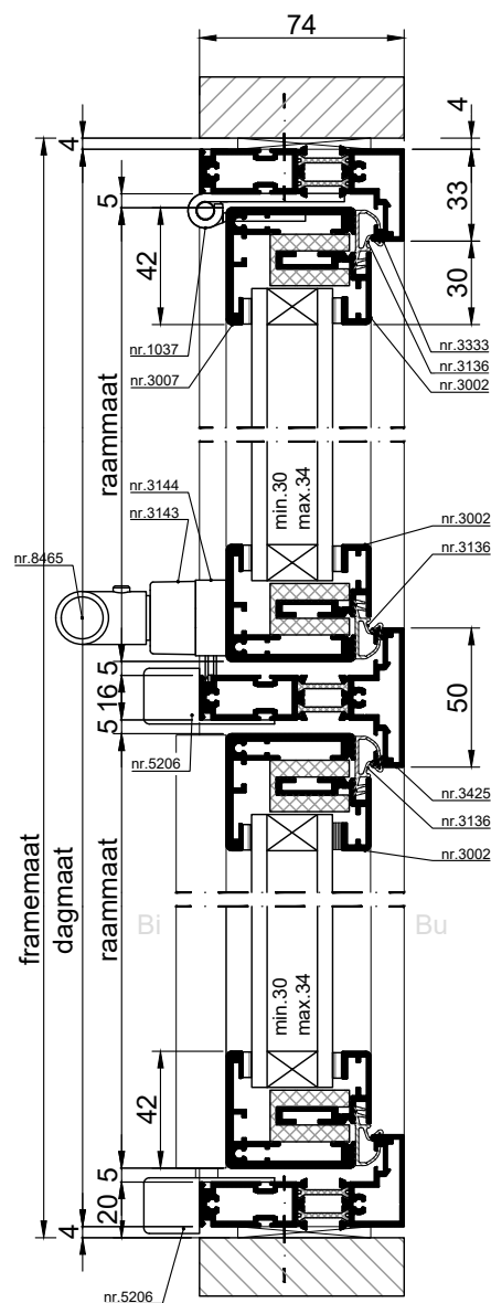
VERTICALE DOORSNEDE type AMC-3
