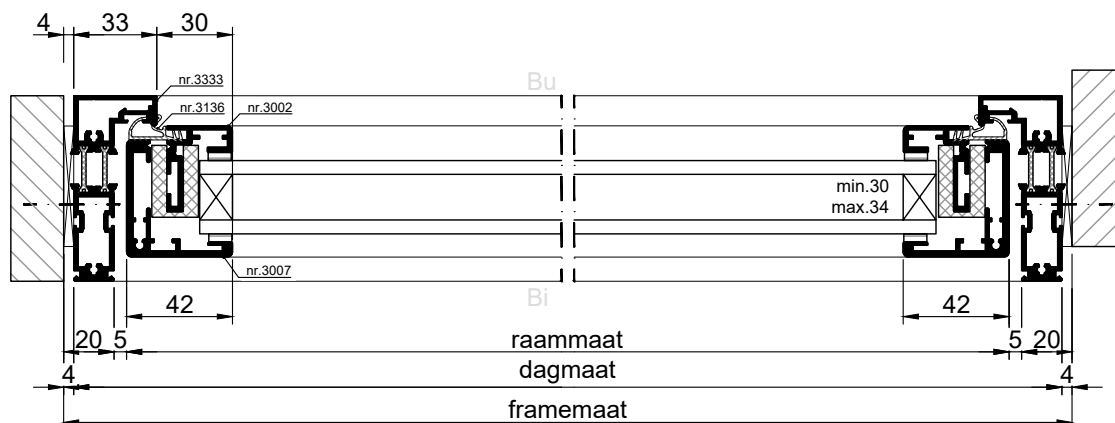
HORIZONTALE DOORSNEDE type AMK-1
