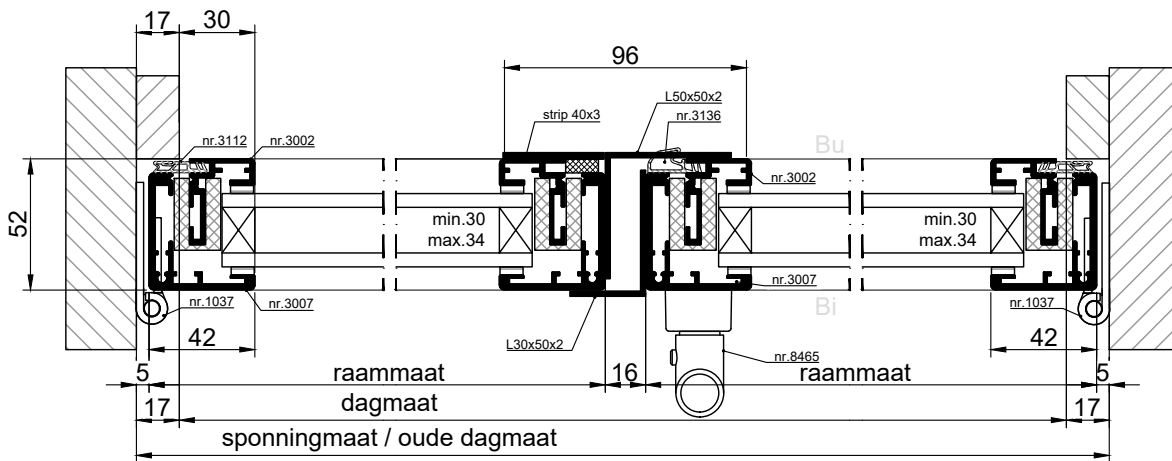
HORIZONTALE DOORSNEDE type AMC-4
