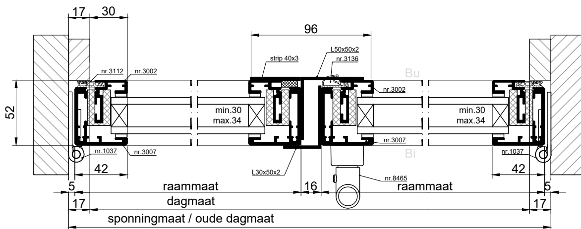
HORIZONTALE DOORSNEDE type AMS-2
