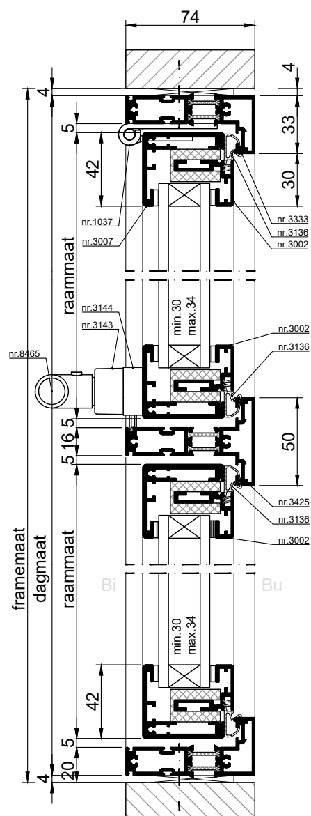
VERTICALE DOORSNEDE type AMC-1
