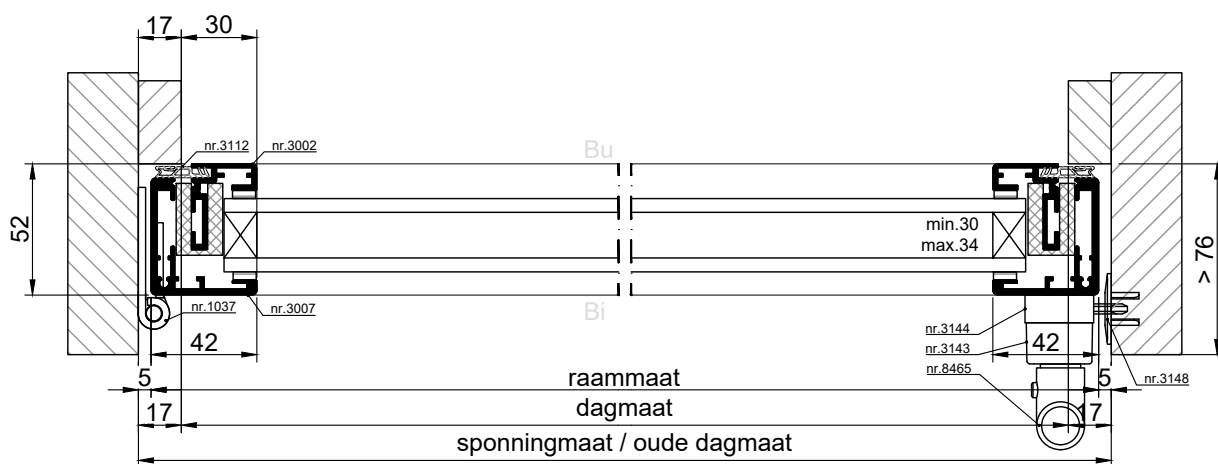
HORIZONTALE DOORSNEDE type AMC-2
