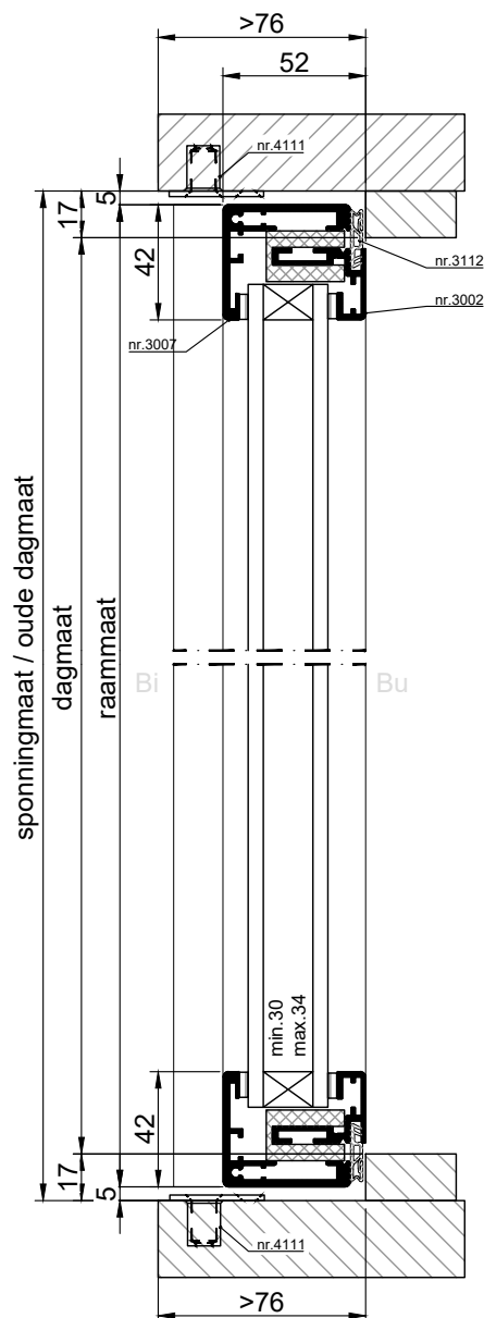
VERTICALE DOORSNEDE type AMS-2
