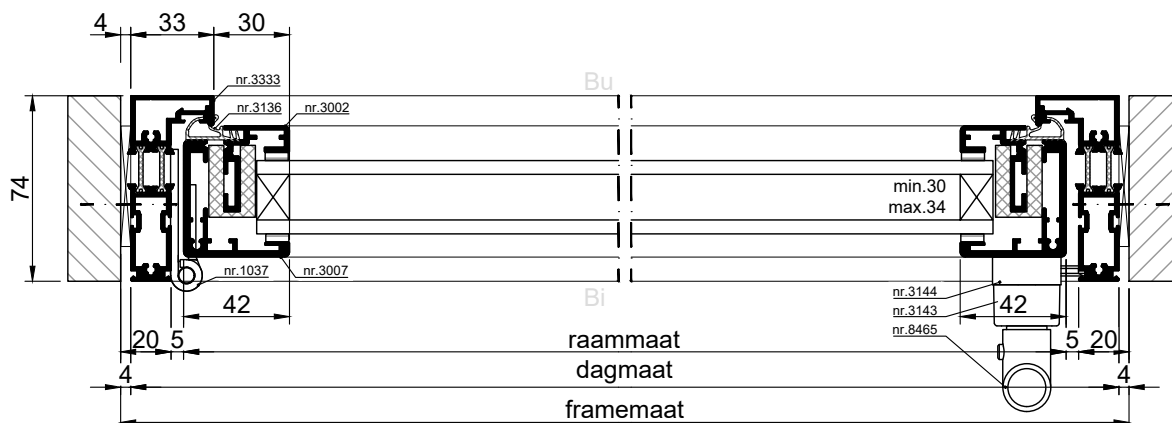
HORIZONTALE DOORSNEDE type AMD-1
