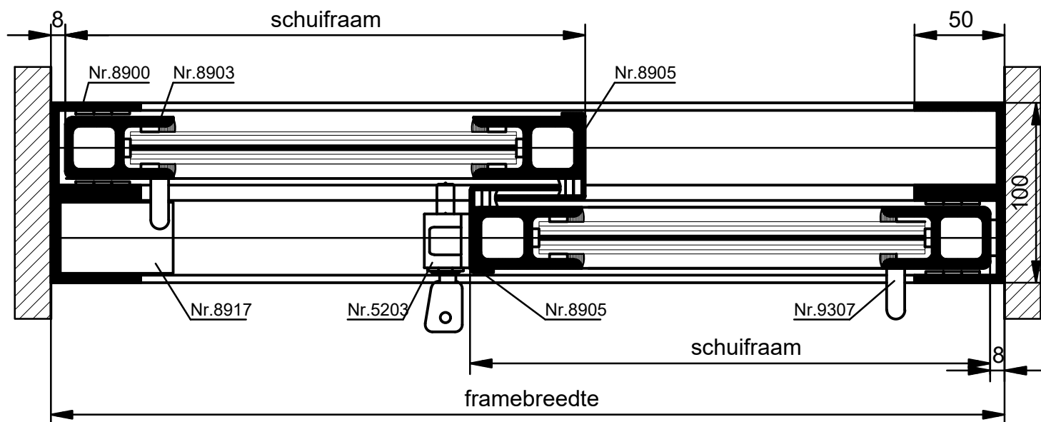
HORIZONTALE DOORSNEDE MHSL-1A
