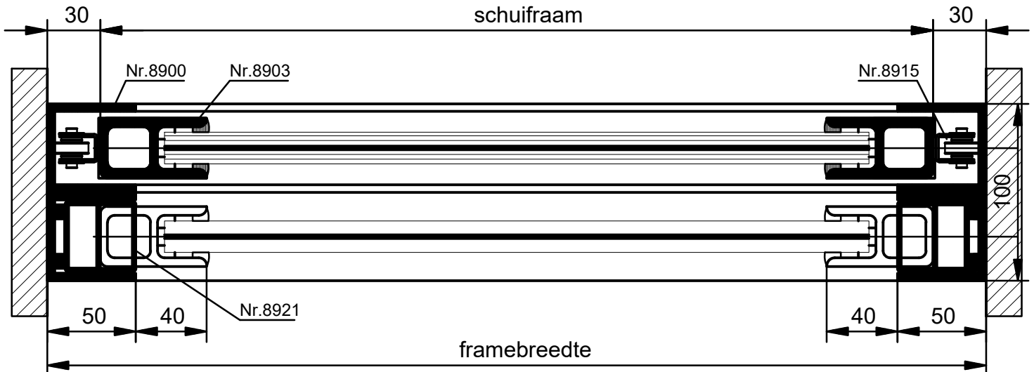
HORIZONTALE DOORSNEDE EMVSL-1A
