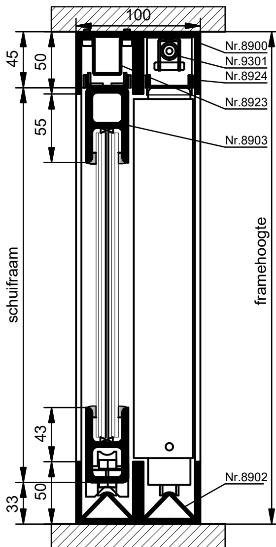
VERTICALE DOORSNEDE MHSL-1E
