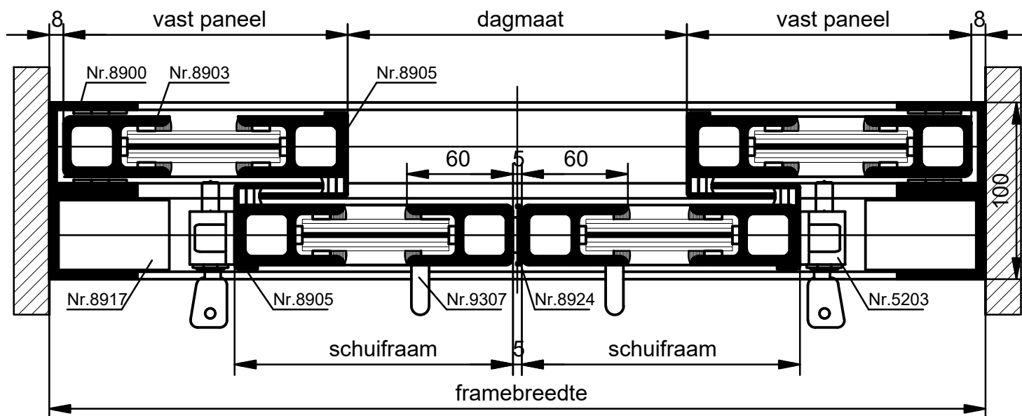
HORIZONTALE DOORSNEDE MHSL-1E
