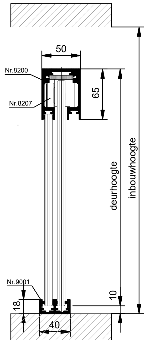
VERTICALE DOORSNEDE type DSD-1
