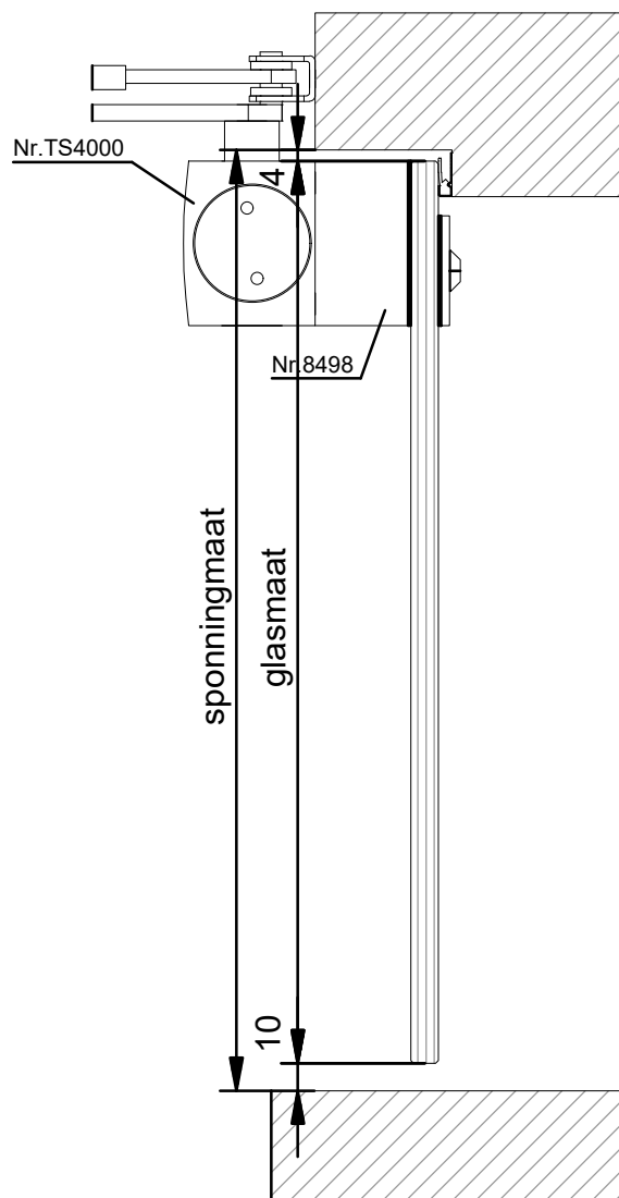
VERTICALE DOORSNEDE type TGD-1C
